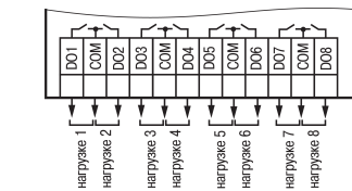
Рисунок 8 – Подключение нагрузки к ВЭ типа «Р»
