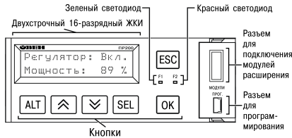
Рисунок 9 – Лицевая панель прибора (крышка отсека подключения модулей условно не показана)
