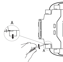
Рисунок 3 – Отсоединение съемных частей клемм
