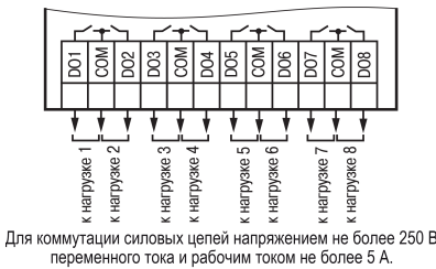
Рисунок 8 – Подключение нагрузки к ВЭ типа «Р»
