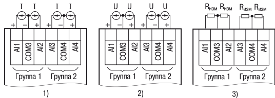
Рисунок 7 – Подключение: 1) активных датчиков с выходом типа «Ток 4...20 мА», 2) активных датчиков с выходом типа «Напряжение 0...10 мВ», 3) датчиков сопротивления с диапазоном 0...4000 Ом
