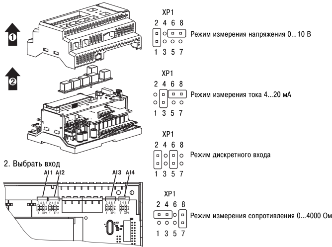
Рисунок 4 – Схема настройки AI1...AI4
