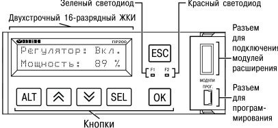
Рисунок 10 – Лицевая панель прибора (крышка отсека подключения модулей условно не показана)
