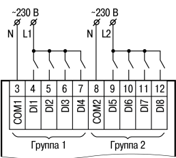
Рисунок 5 – Подключение дискретных датчиков с питанием 230 В
