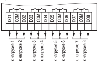
Рисунок 6 – Подключение нагрузки к ВЭ типа «Р»
