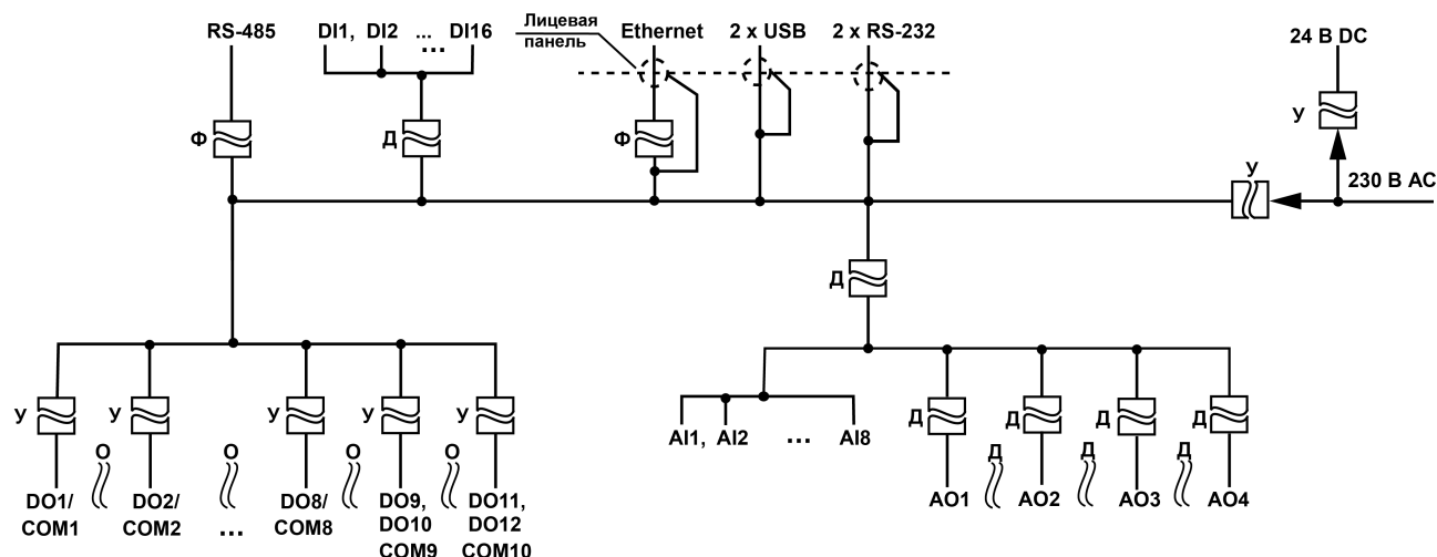
Рисунок 2.1 – Схема электрической прочности изоляции ПЛК160-220.X-M(М02)
