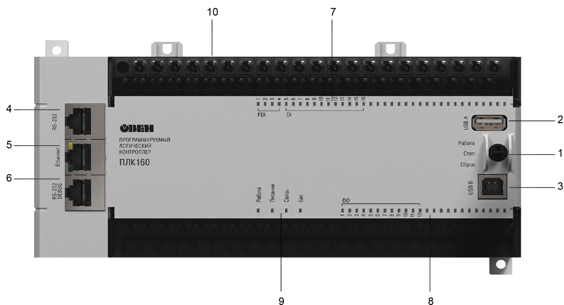
Рисунок 3.1 – Внешний вид ПЛК160(М02)
