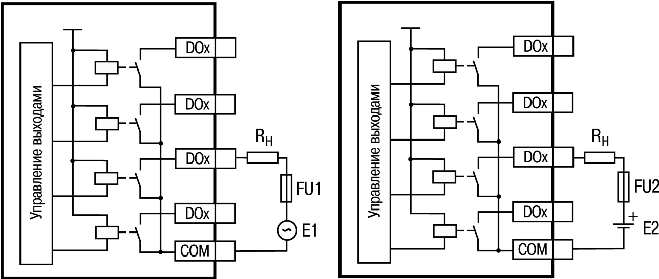
Рисунок 6.12 – Выходные элементы типа Р с внешними цепями защиты при активной нагрузке, R н – пользовательская нагрузка (двигатель, нагреватель, контактор и т. д.)
