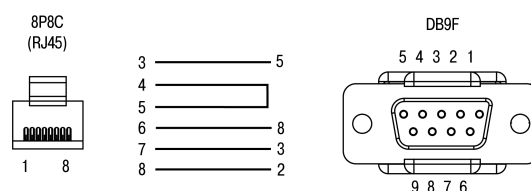
Рисунок 6.13 – Схема кабеля программирования KC14, входящего в комплект поставки
