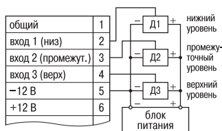
Подключение активных датчиков Д1...Д3 при питании их от внешнего источника
