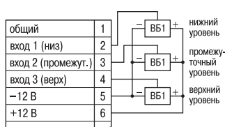
Подключение емкостных переключателей
