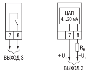
ВЭ3 типа Р (э/м реле)
