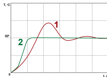
Работа регулятора в режиме автонастройки
