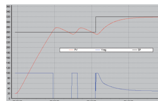
Работа регулятора в режиме автонастройки
