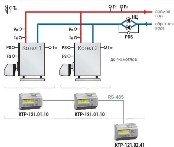
Для каскада до 4-х котлов с регулированием общей температуры обратной воды КЗР
