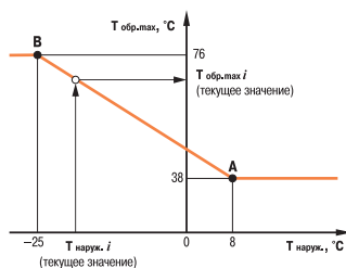
Пример графика температуры обратной воды — T_{обр.мах} = f(T_{нарук.})
