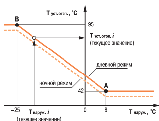
Пример отопительного графика — T_{уст.отоп.} = f(T_{нарук.})
