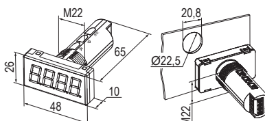
Щ9 48×26×65 мм IP54
