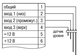
Подключение кондуктометрических датчиков уровня
