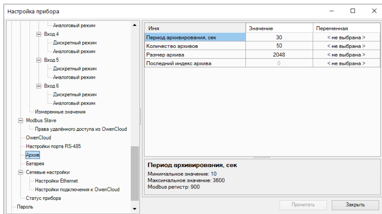
Рисунок 4.17 – Настройка параметров архива
