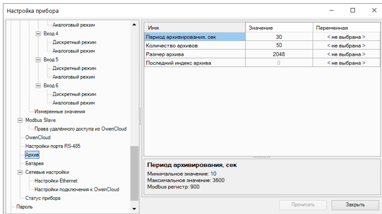
Рисунок 4.10 – Настройка параметров архива
