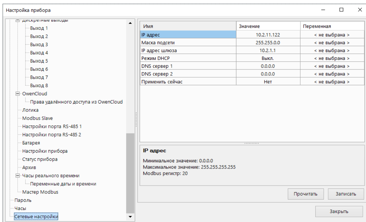
Рисунок 4.18 – Настройки параметров Ethernet
