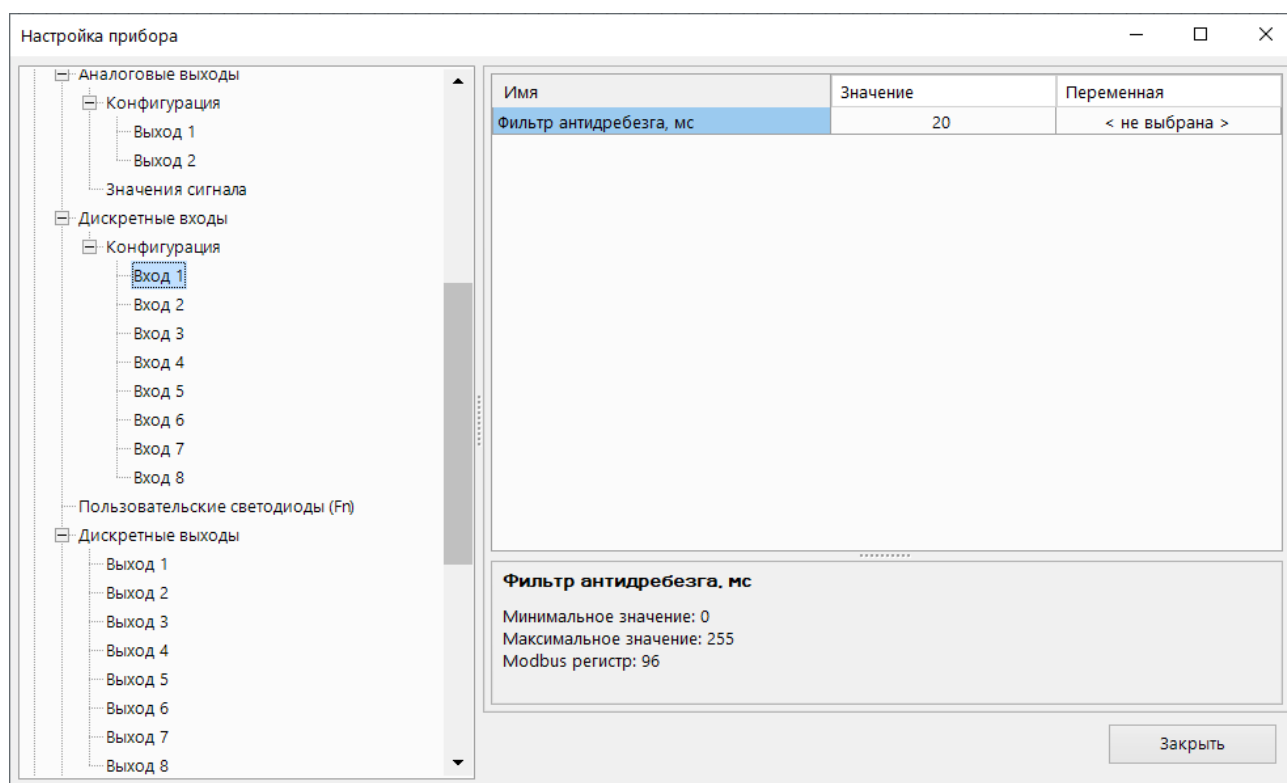
Рисунок 4.8 – Настройка фильтра дискретного входа
