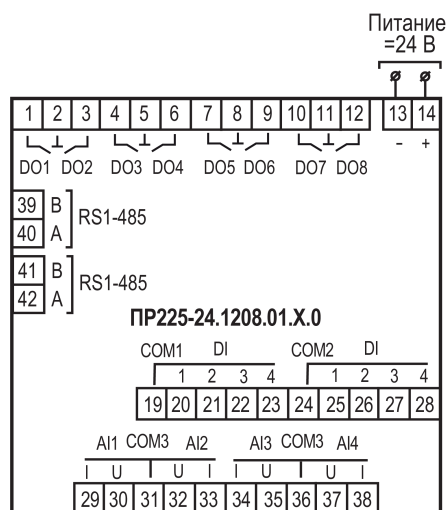
Рисунок А.6 – Расположение контактов для PR225–24.1208.01.X.0
