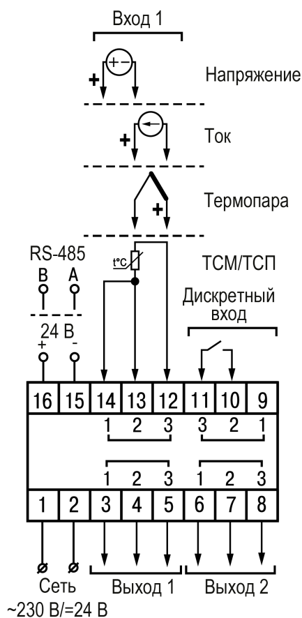
Рисунок 5.5 – Общая схема подключения ТРМ10–Щ5
