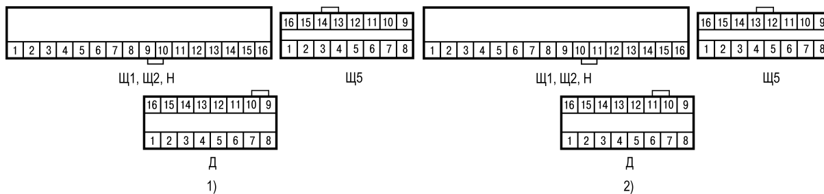
Рисунок 7.9 – Установка перемычки
