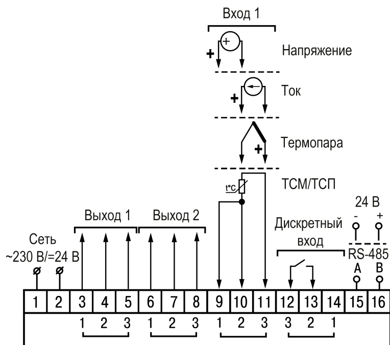
Рисунок 5.7 – Общая схема подключения TPM10–Н
