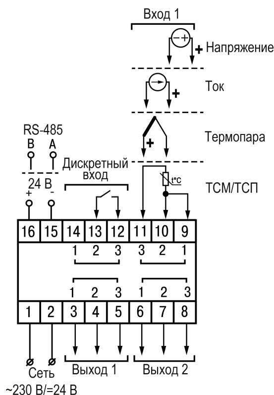
Рисунок 5.6 – Общая схема подключения TPM10–Д
