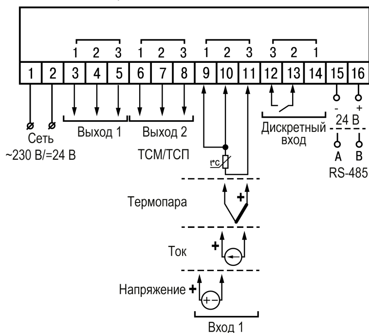
Рисунок 5.4 – Общая схема подключения ТРМ10–Щ1/Щ2
