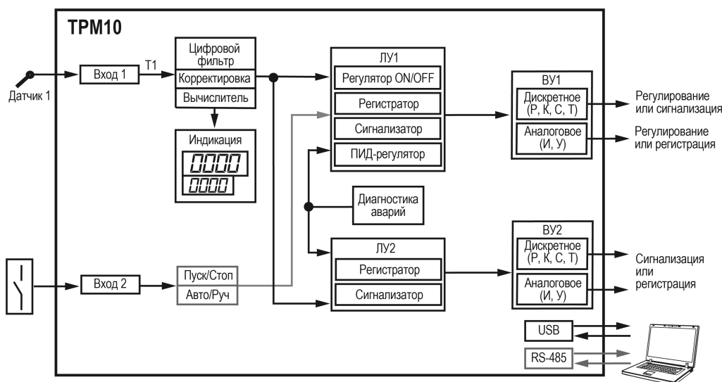
Рисунок 6.1 – Функциональная схема
