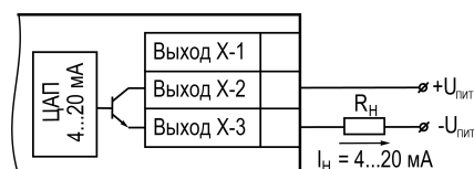
Рисунок 5.27 – Подключение к ВУ типа «И»
