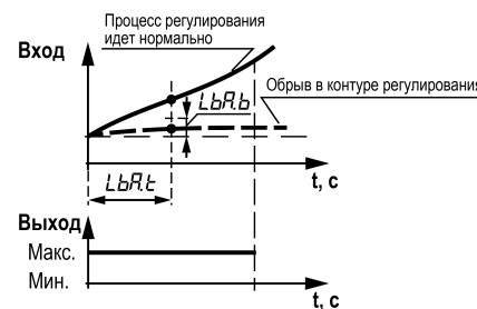
Рисунок 7.4 – Диагностика неисправности контура регулирования
