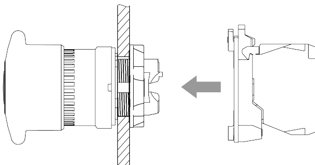
Рисунок 6.4 – Завершение монтажа
