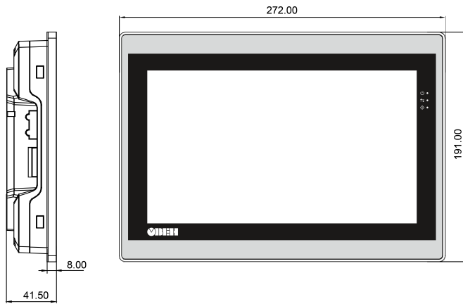
Рисунок 1 – Габаритные размеры прибора
