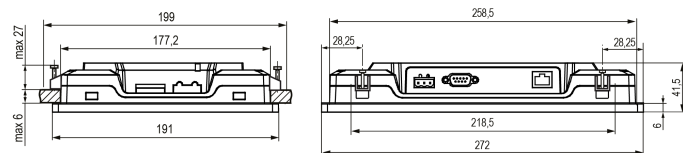
Рисунок 3 – Дополнительные установочные размеры прибора
