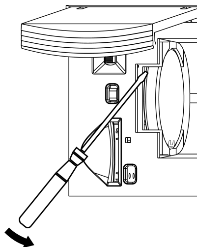
Рисунок 3.6 – Извлечение батареи
