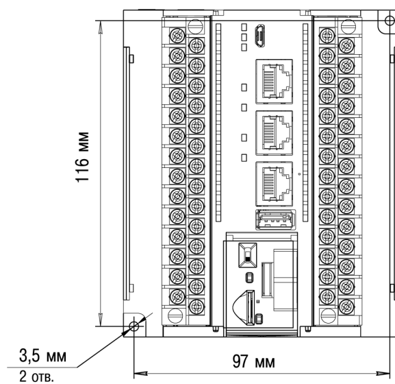
Рисунок 4.3 – Монтажные размеры
