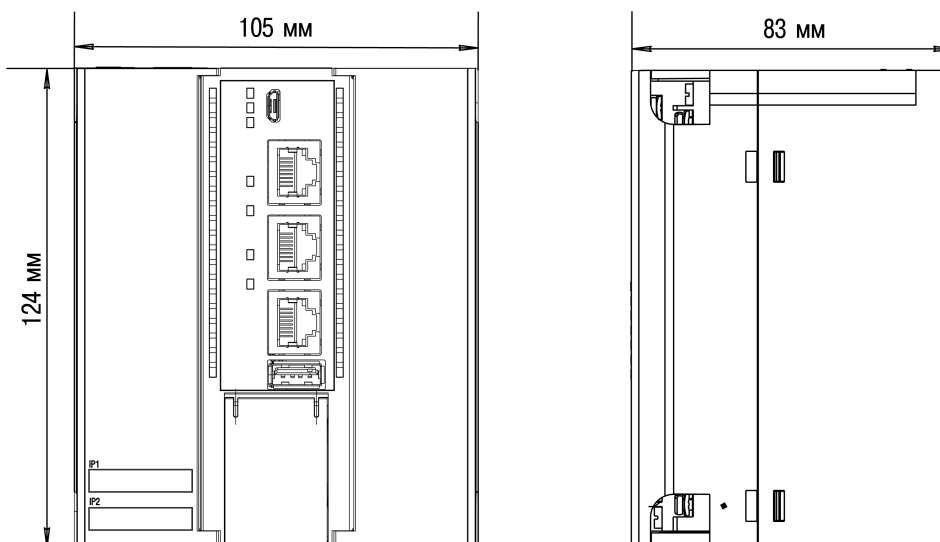
Рисунок 4.2 – Габаритные размеры
