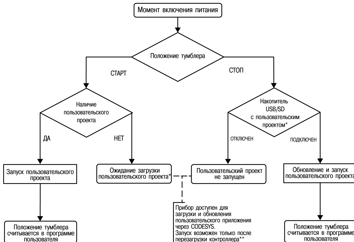
Рисунок 3.5 – Принцип работы тумблера
