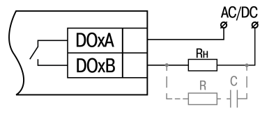
Рисунок 14 – Схема подключения нагрузки к дискретным выходам типа «реле»
