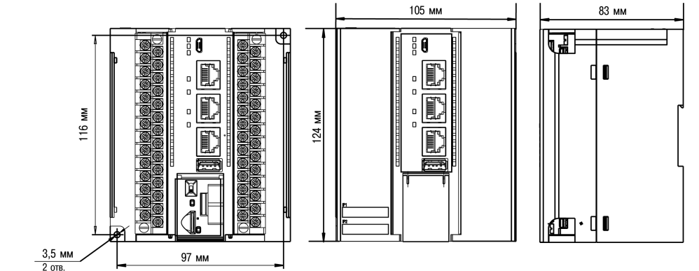
Рисунок 1 – Габаритные и монтажные размеры
