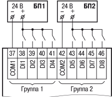
Рисунок 4 – Подключение дискретных датчиков с питанием 24 В
