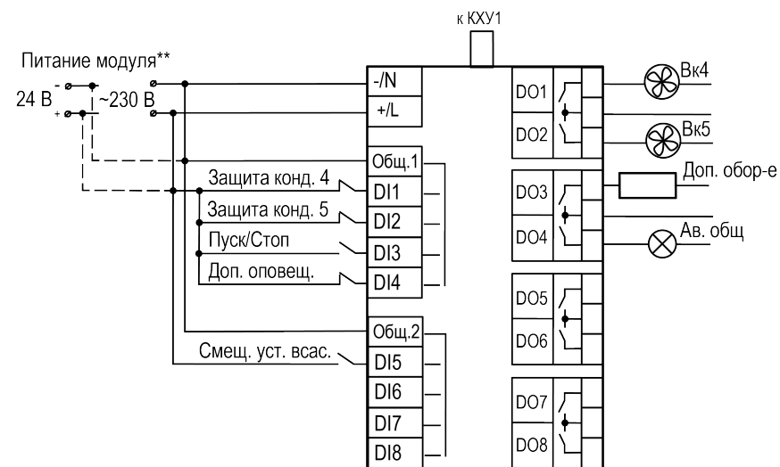
Рисунок 7.12 – Пример схемы подключения пяти компрессоров, пяти вентиляторов с индивидуальными сигналами защиты, дистанционный пуск по кнопке, сигнал дополнительного аварийного оповещения, сигнал для смещения уставки всасывания, функция Термостат, реле аварии
