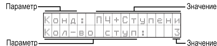
Рисунок 6.2 – Внешний вид параметра и значения на ЖКИ
