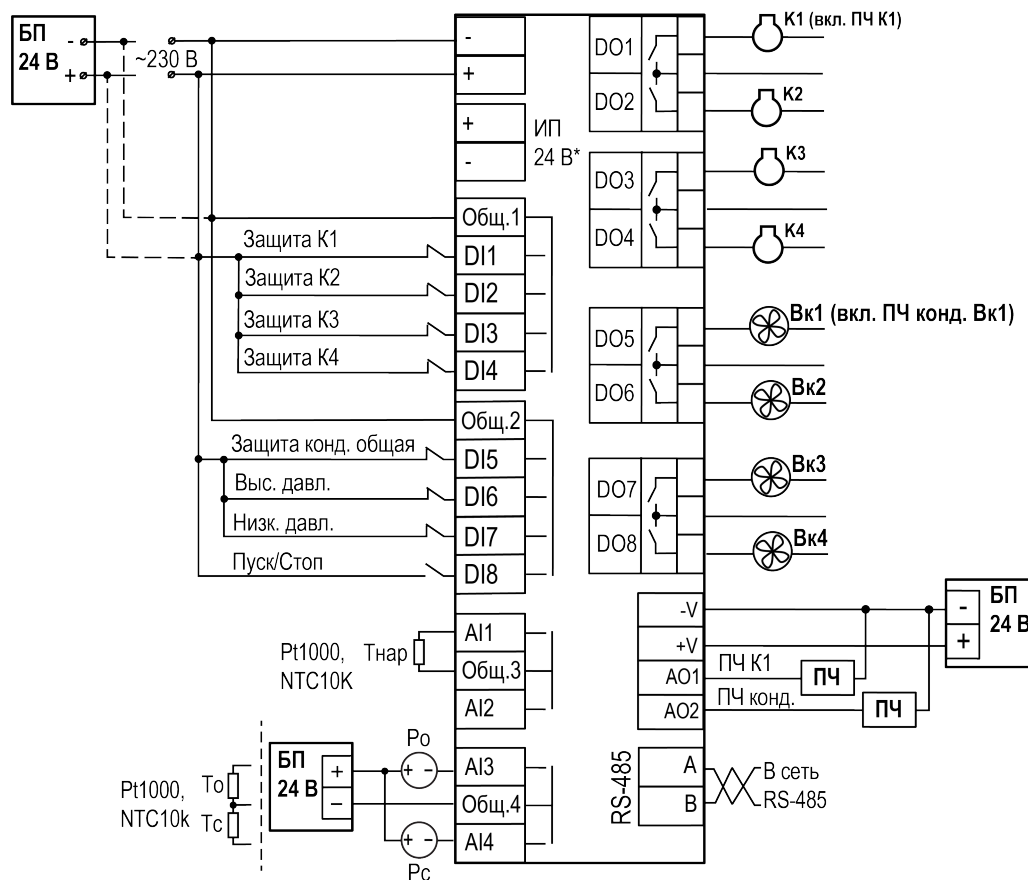
Рисунок 7.11 – Пример схемы подключения четырех компрессоров, четырех вентиляторов с общим сигналом защиты, реле общего высокого и низкого давления, дистанционный пуск по кнопке
