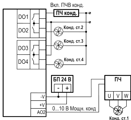
Рисунок 7.9 – Схема подключения на примере конфигурации из 4-х ступеней конденсатора, где 1-я ступень управляется ПЧ, без компрессоров
