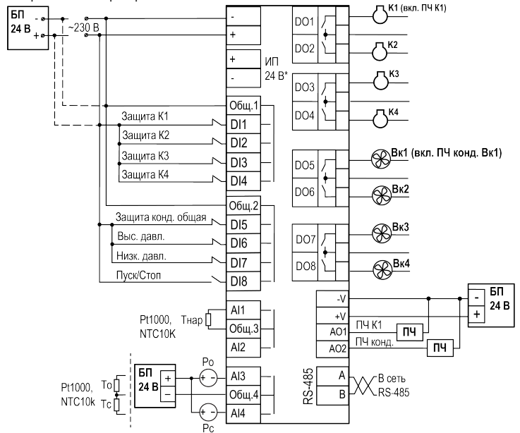
Рисунок 3 – Схема подключения сигналов
