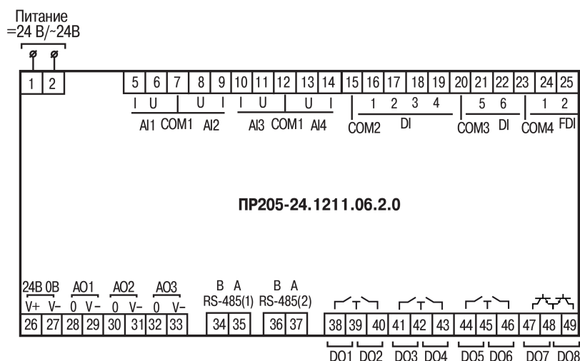
Рисунок А.8 – Расположение контактов для ПР205-24.1211.06.2.0
