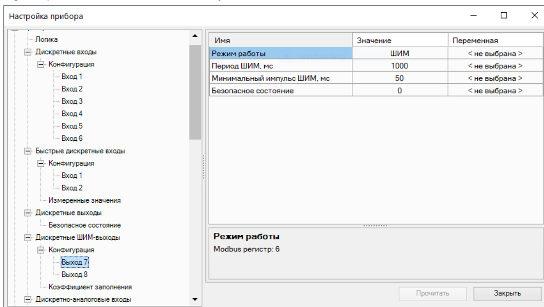
Рисунок 4.16 – Настройка параметров работы выхода типа «КТ» в режиме ШИМ
