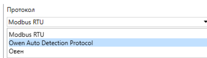
Рисунок 4.18 – Выбор протокола
