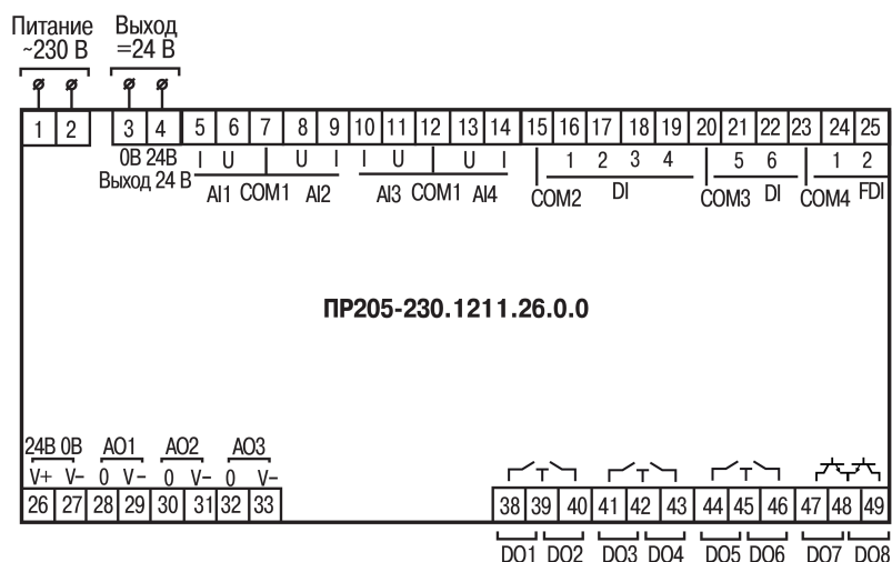
Рисунок А.3 – Расположение контактов для PR205-230.1211.26.0.0
