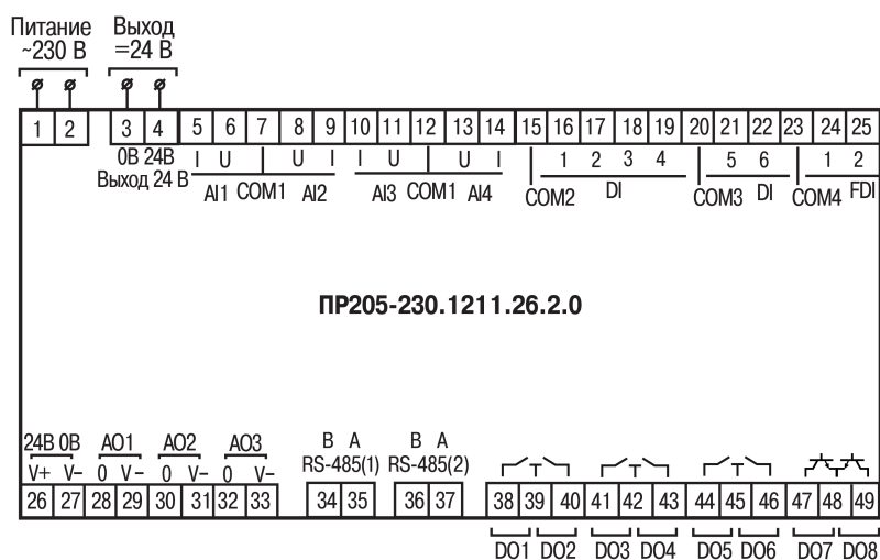
Рисунок А.4 – Расположение контактов для PR205-230.1211.26.2.0
