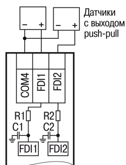
Рисунок 6.2 – Подключение к входам типа «ДС» датчиков с выходом push-pull
