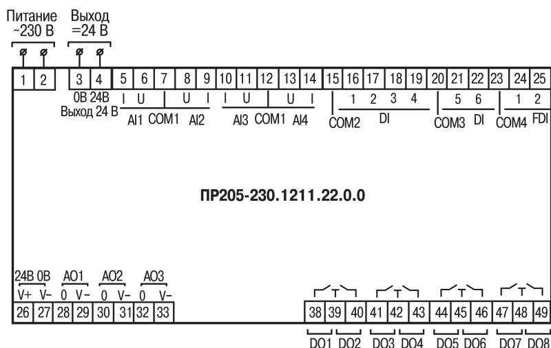
Рисунок А.1 – Расположение контактов для ПР205-230.1211.22.0.0
