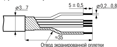
Рисунок 5.5 – Подготовка кабеля
