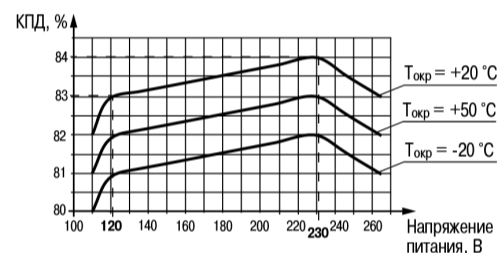
Рисунок 8 – График зависимости КПД от напряжения питания и температуры окружающей среды (с учетом АКБ)
