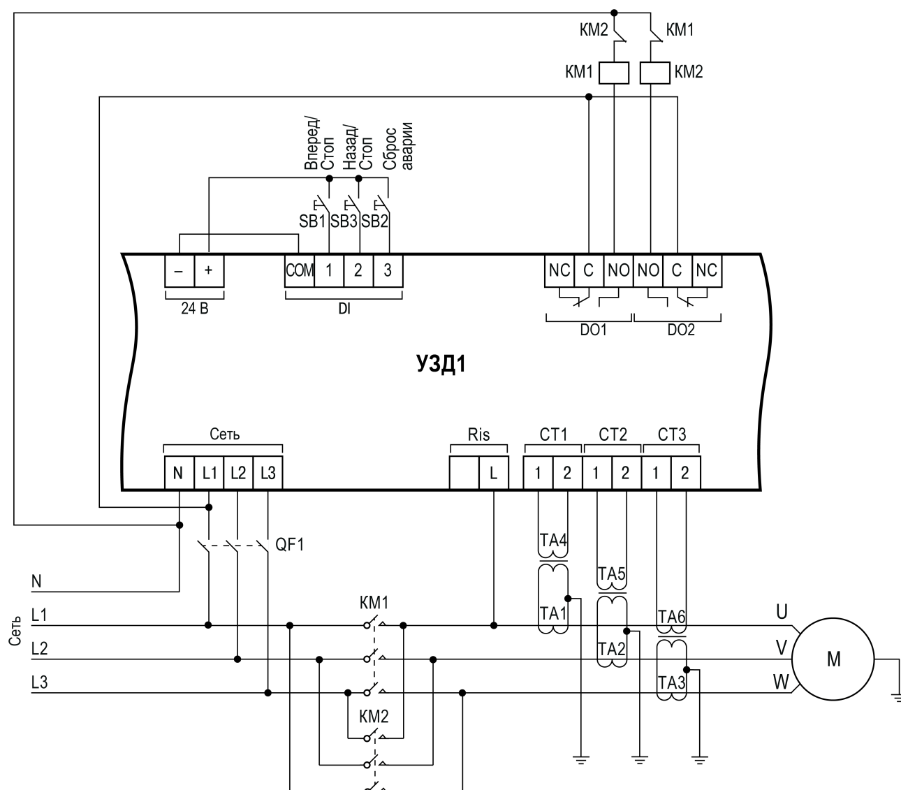
Рисунок 5.3 – Электрическая схема реализации реверсивного режима работы электродвигателя
