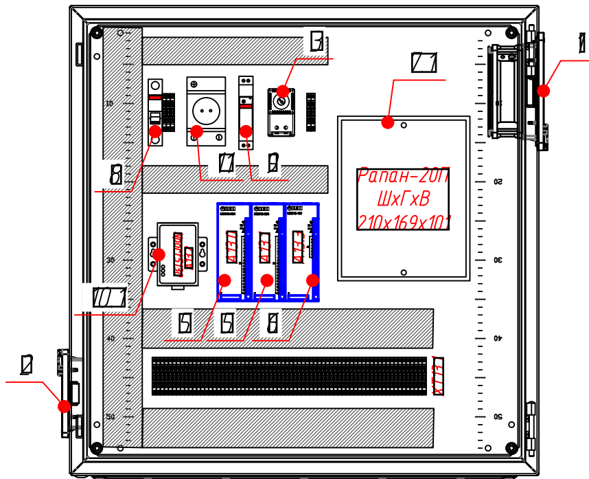
Вид спереди (дверь не показана)
