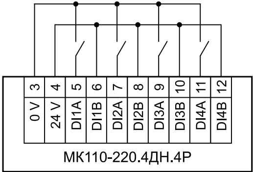
Рисунок 3 – Подключение контактных датчиков (питание от встроенного источника)
