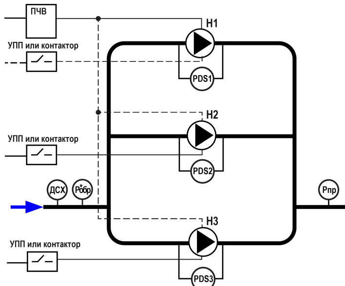
Рисунок 6.1 – Объект управления
