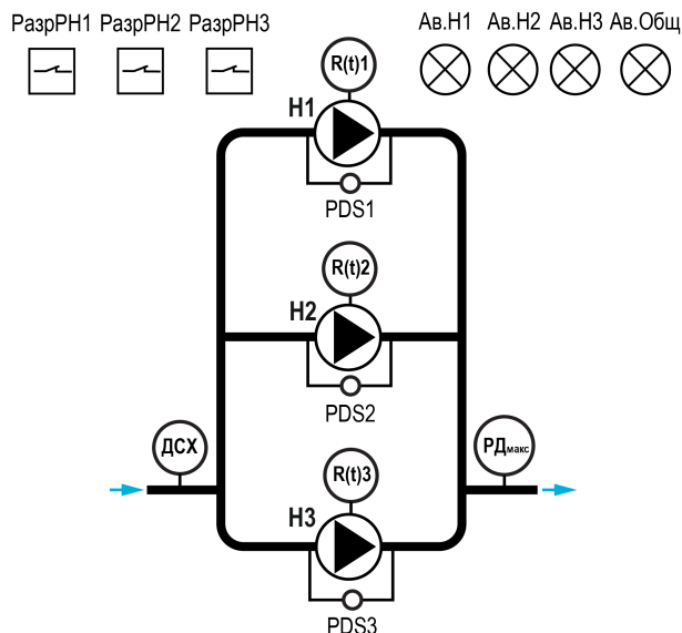
Рисунок 7.1 – Объект управления
