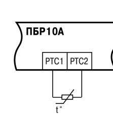
Рисунок 6 – Схема подключения PTC-датчика
