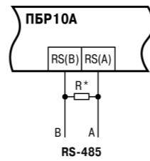
Рисунок 5 – Схема подключения интерфейса RS-485
