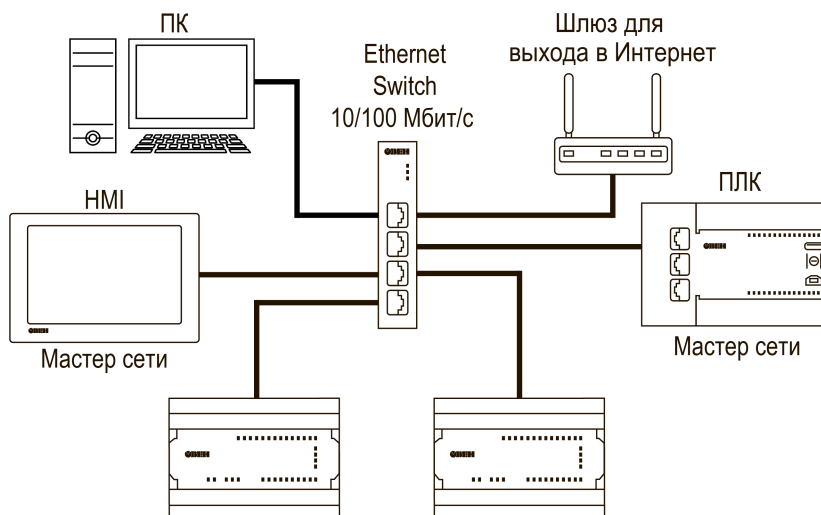
Рисунок 6.23 – Подключение по схеме «Звезда»
