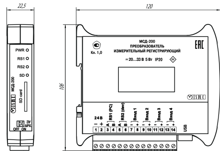
Рисунок 2 – Габаритные размеры
