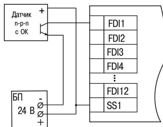
Рисунок 5.9 – Подключение транзисторов типа н-п-п* к дискретным входам FDI1–FDI12
