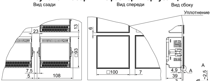
Рисунок 6 – Габаритные размеры корпуса Щ11
