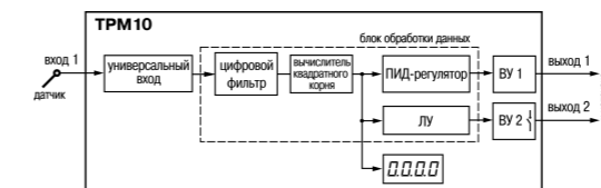
Рисунок 28 – Функциональная схема прибора
