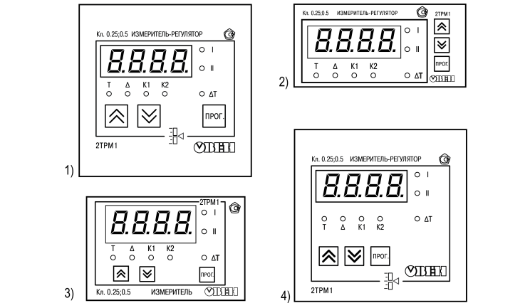
Рисунок 28 – Лицевая панель прибора для корпусов: 1) настенного Н и щитового крепления Щ1; 2) щитового Щ2; 3) DIN-реечного Д; 4) щитового Щ11
