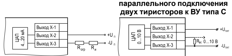
Рисунок 24 – Схема встречно-параллельного подключения двух тиристоров к ВУ типа С
