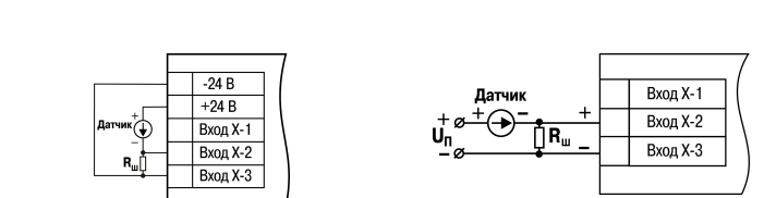
Рисунок 16 – Схема подключения активного датчика с выходом в виде напряжения от -50 до 50 мВ или от 0 до 1 В
