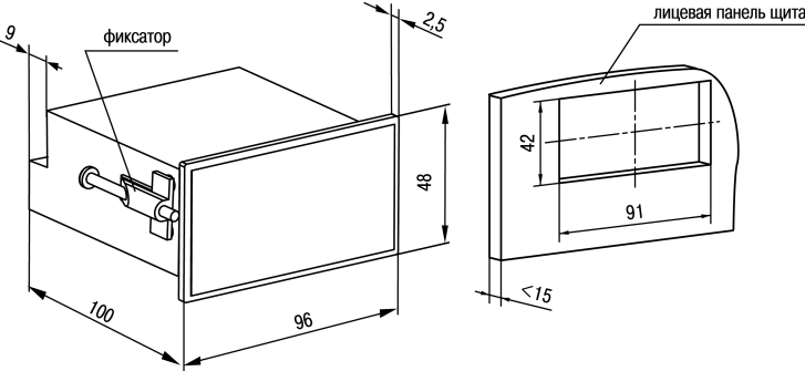
Рисунок 4 – Габаритные размеры корпуса Щ2
