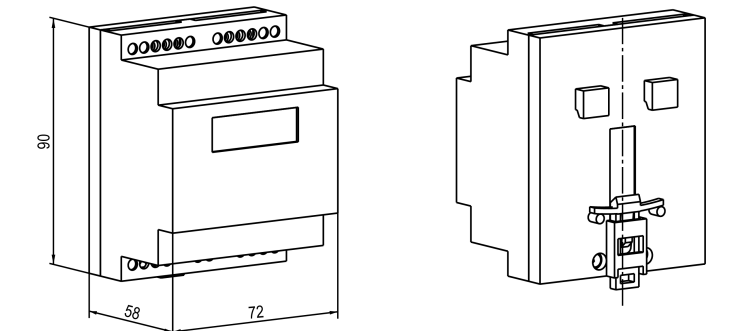
Рисунок 9 – Габаритные размеры корпуса Д
