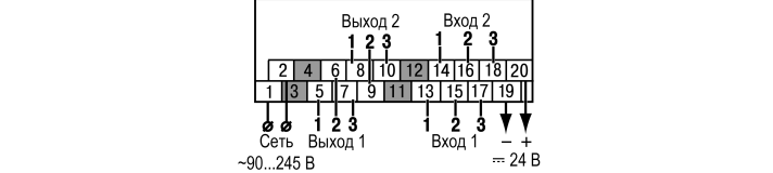
Рисунок 11 – Назначение контактов клеммной колодки прибора в корпусе Щ11
