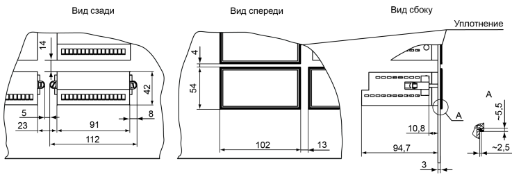
Рисунок 5 – Прибор в корпусе Щ2, установленный в щит толщиной 3 мм
