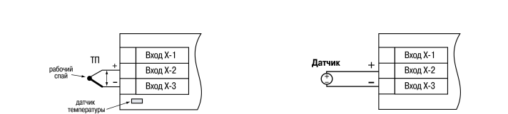
Рисунок 14 – Двухпроводная схема подключения ТС
