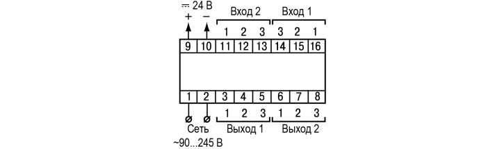
Рисунок 12 – Назначение контактов клеммной колодки прибора в DIN-реечном Д корпусе
