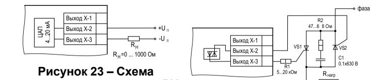
Рисунок 23 – Схема подключения нагрузки к ВУ типа И
