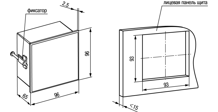
Рисунок 2 – Габаритные размеры корпуса Щ1
