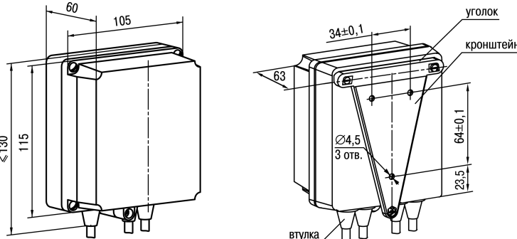
Рисунок 1 – Габаритные размеры корпуса Н
