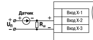
Рисунок 17 – Схема подключения пассивного датчика с токовым выходом от 0 до 5 мА или от 0(4) до 20 мА R_{ш} = 49,9 \pm 0,025 \text{ Ом}
