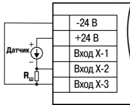
Рисунок 18 – Схема подключения пассивного датчика с питанием от прибора
