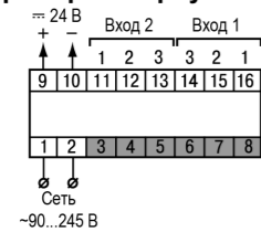
Рисунок 12 – Назначение контактов клеммной колодки прибора в DIN-реечном Д корпусе
