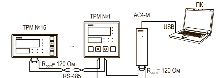
Рисунок 30 – Подключение приборов по сети RS-485
