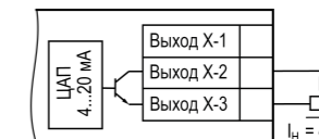
Рисунок 26 – Подключение к ВУ типа «И»
