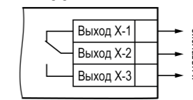
Рисунок 22 – Схема подключения нагрузки к ВУ типа «Р»
