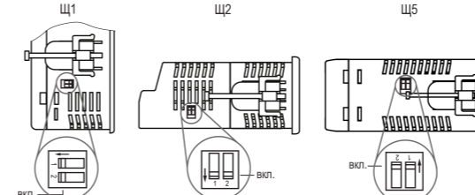
Рисунок 20 – Расположение DIP-переключателей
