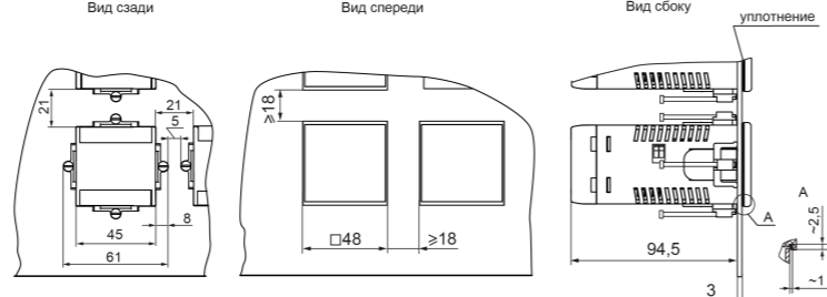
Рисунок 9 – Корпус Щ5 в щите толщиной 3 мм
