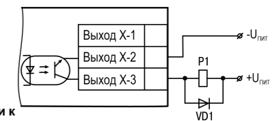
Рисунок 23 – Схема подключения нагрузки к ВУ типа «К»
