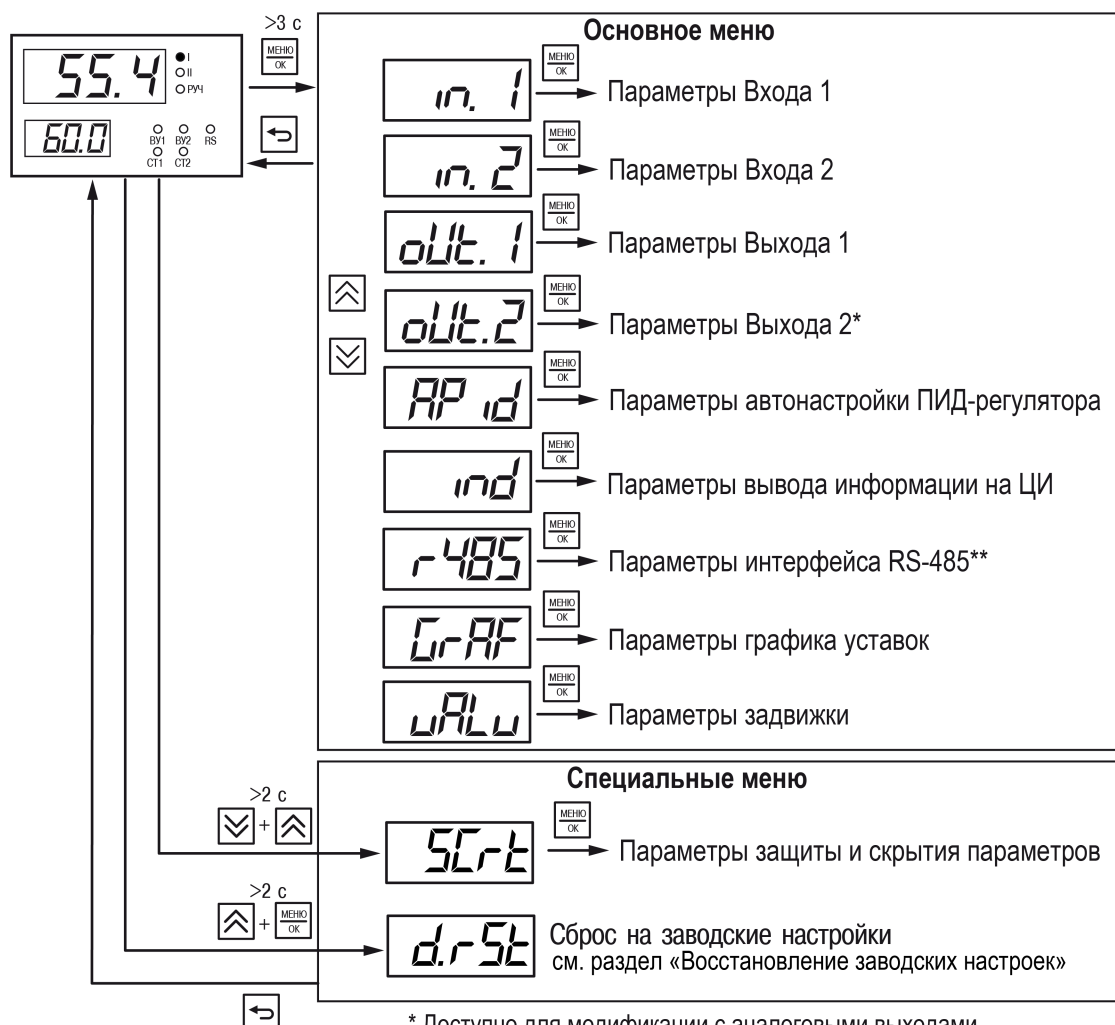
Рисунок 7.1 – Структура меню
