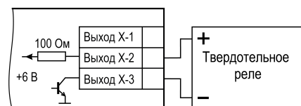
Рисунок 5.18 – Схема подключения нагрузки к ВУ типа «Т»
