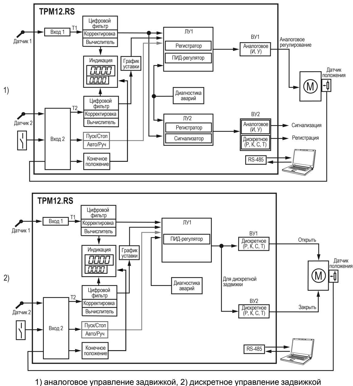
Рисунок 6.1 – Функциональная схема
