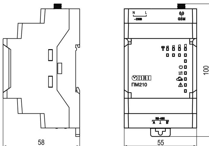
Рисунок 4.1 – Габаритные размеры
