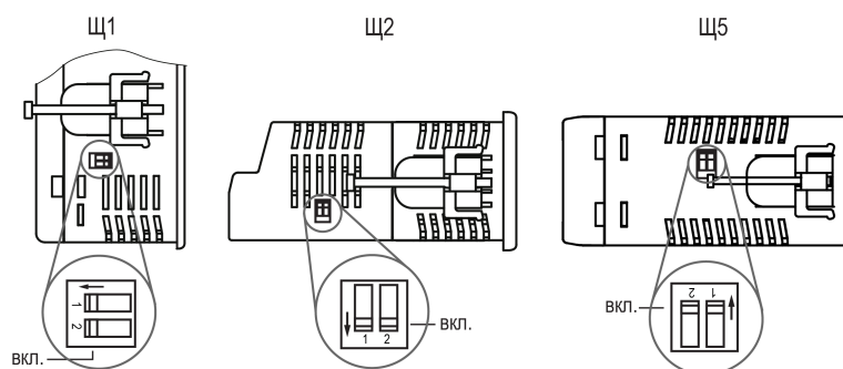
Рисунок 5.14 – Расположение DIP-переключателей
