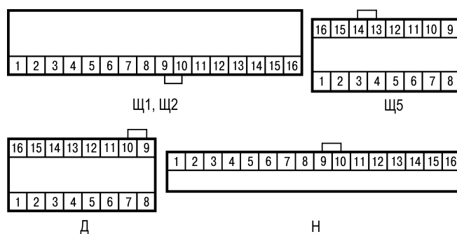
Рисунок 7.6 – Установка перемычки
