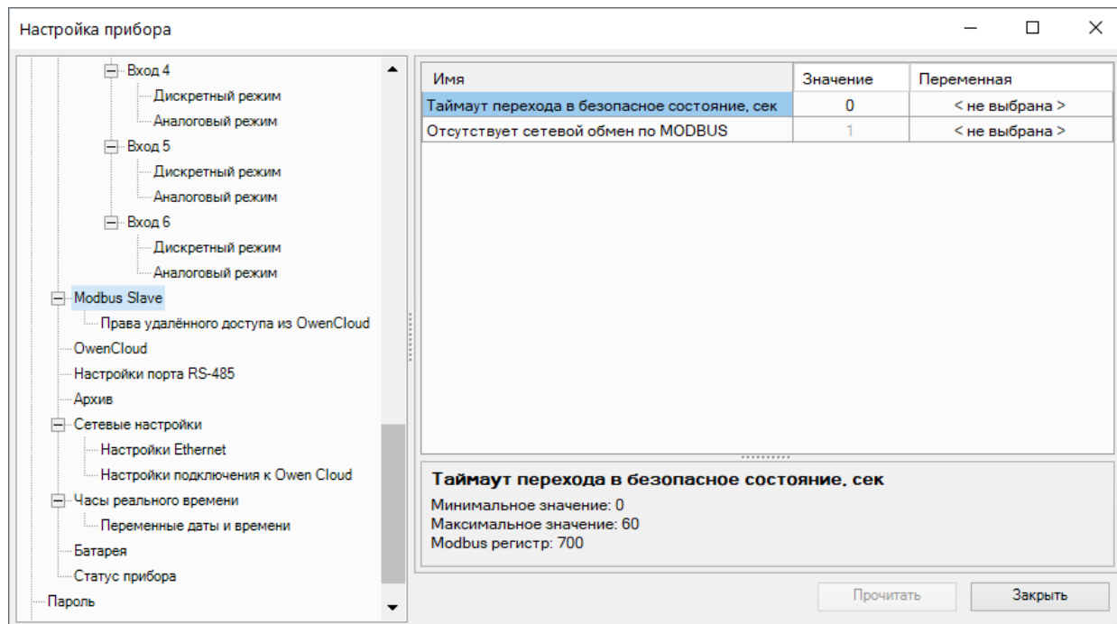
Рисунок 4.22 – Настройка работы по протоколу Modbus TCP в OwenLogic
