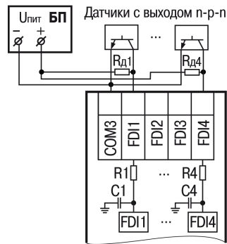
Рисунок 6.7 – Подключение к входам типа «ДС» датчиков с выходом п-р-п
