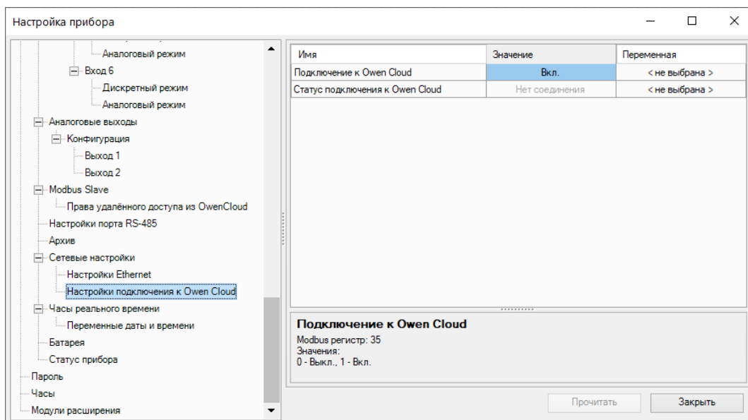
Рисунок 4.23 – Настройки подключения к OwenCloud
