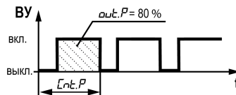
Рисунок 7.4 – Мощность дискретного ВУ
