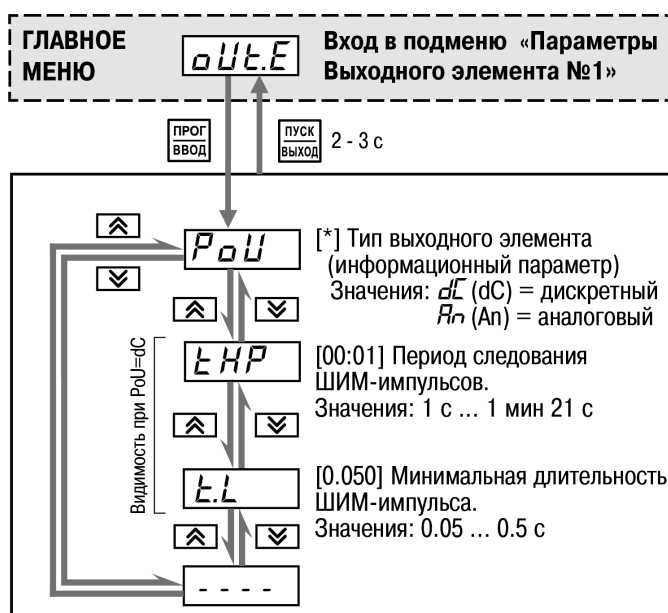
Рисунок 8.7 – Параметры ВЭ1
