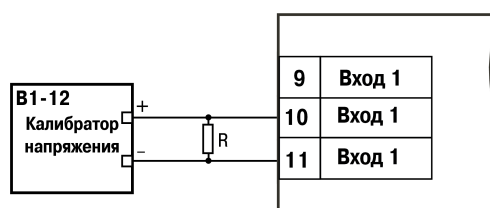
Рисунок 11.4 – Подключение калибратора напряжения 2
