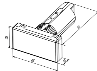
Рисунок 4.2 – Габаритные размеры корпуса щита
