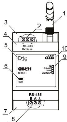
Рисунок 2 – Общий вид прибора
