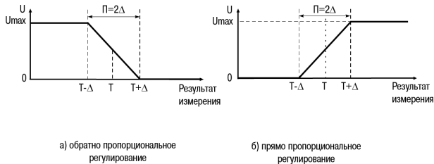
Рисунок 7.9 – Принцип формирования выходного сигнала П-регулятора для приборов с ВУ типа А
