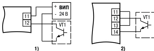
Рисунок 5.3 – Подключение дискретных датчиков с п-п-выходом: 1) при работе датчика от ВИП; 2) при работе датчика от внутреннего источника питания
