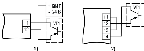
Рисунок 5.4 – Подключение дискретных датчиков с п-п-выходом: 1) при работе датчика от ВИП; 2) при работе датчика от внутреннего источника питания
