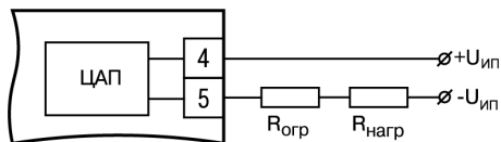
Рисунок 5.5 – Схема подключения ВУ типа И
