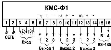
Рисунок 5.1 – Назначение клеммника
