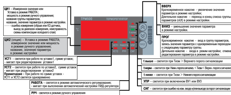
Рисунок 5 – Назначение ЦИ, кнопок и светодиодов
