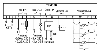
Рисунок 3 – Общая схема подключения
