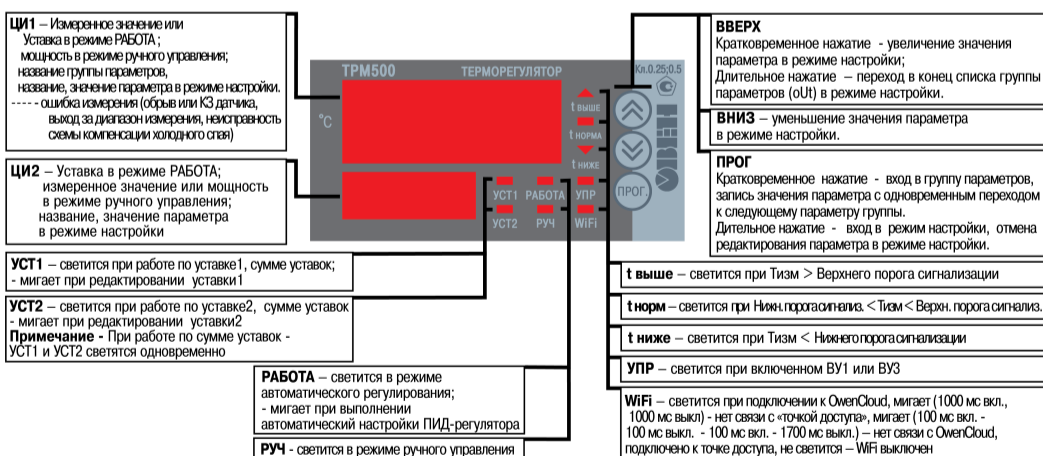
Рисунок 5 – Назначение ЦИ, кнопок и светодиодов
