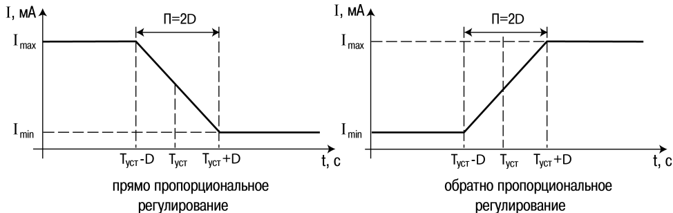
Рисунок 7.8 – Виды регулирования
