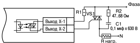
Рисунок 5.14 – Схема подключения силового симистора к ВУ типа С
