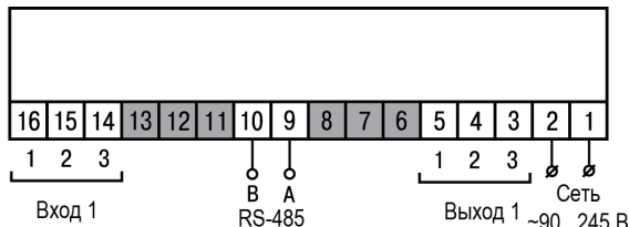
Рисунок 5.3 – Общая схема подключения TRM201-H2
