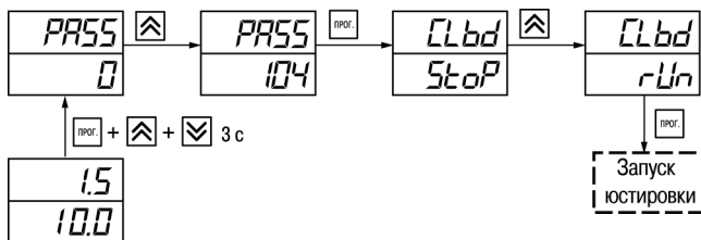
Рисунок 8.2 – Запуск юстировки
