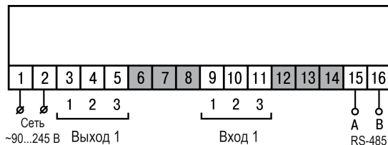
Рисунок 5.2 – Общая схема подключения TRM201-H, -Щ1 и -Щ2
