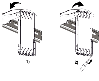
Рисунок 6.2 – Монтаж (1) и демонтаж (2) прибора
