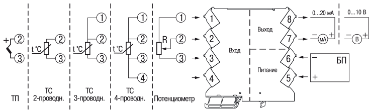
Рисунок 6.3 – Подключение прибора
